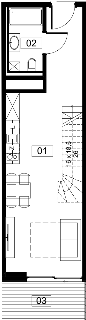
POZIOM I ( 36,96 m 2 )
