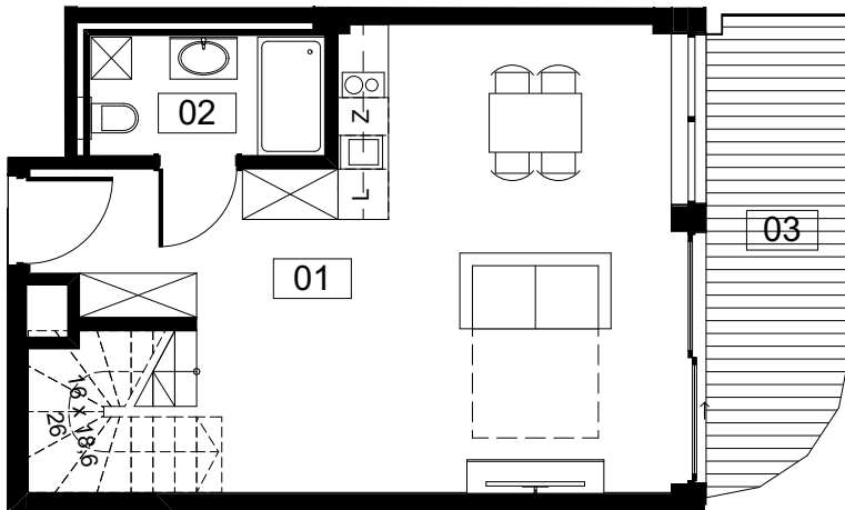
POZIOM I ( 40,53 m 2 )
