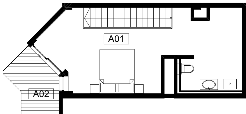
POZIOM II (27,70 m 2 )
