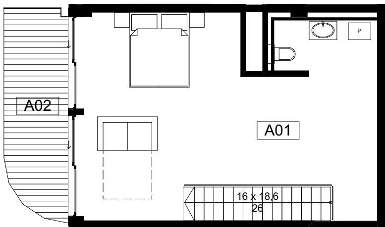
POZIOM II (39,87 m 2 )
