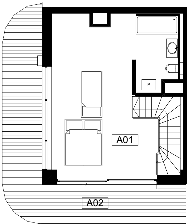
POZIOM II (35,20 m 2 )
