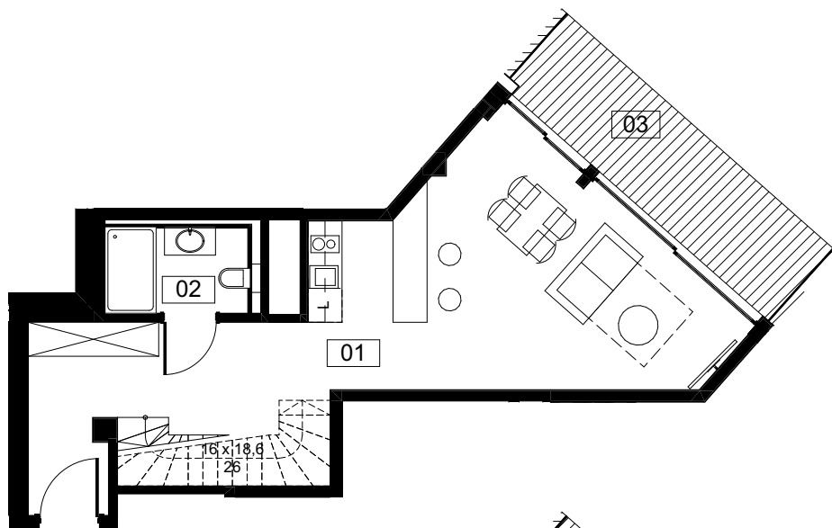
POZIOM I ( 44,80 m 2 )
