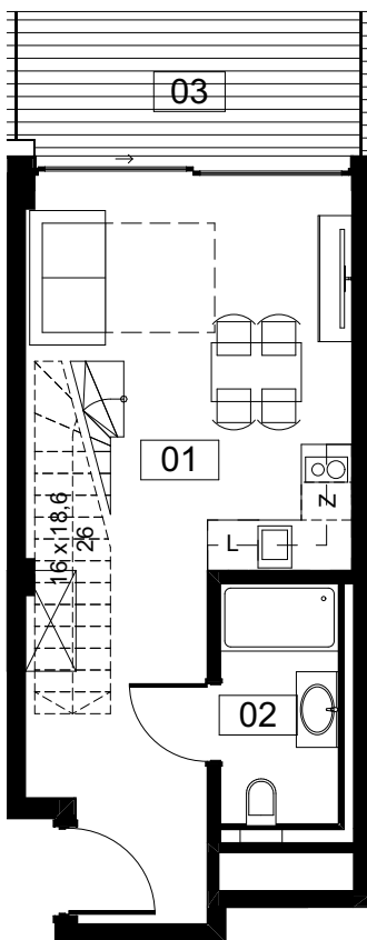
POZIOM I ( 30,00 m 2 )
