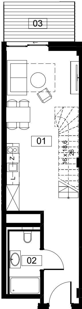
POZIOM I ( 35,94 m 2 )
